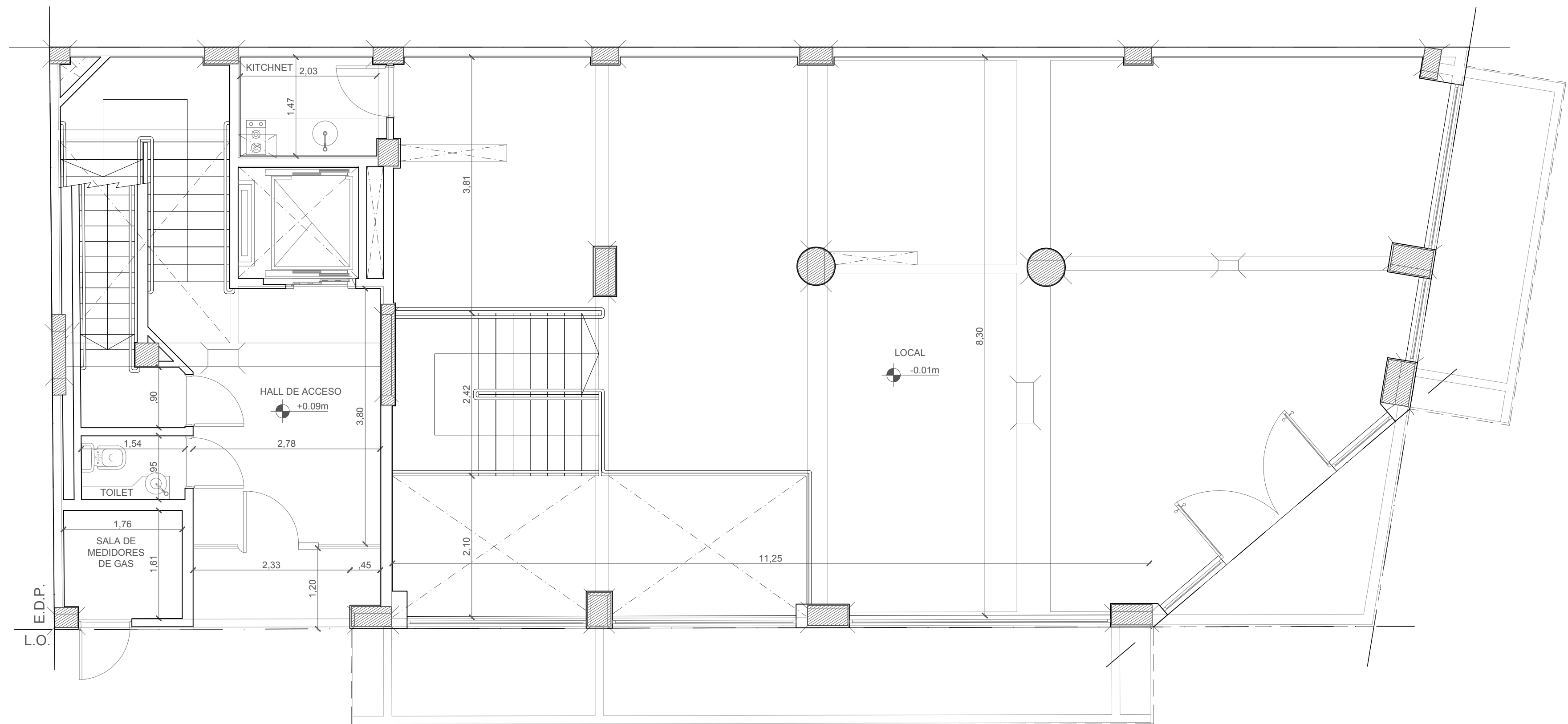
PLANTA BAJA
