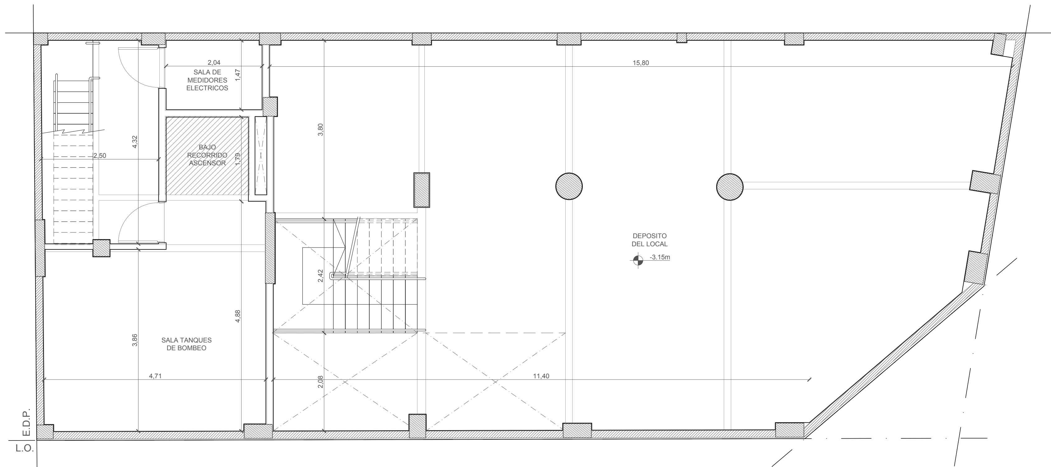
PLANTA SUBSUELO
